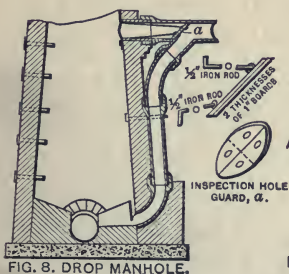
FIG. 8. DROP MANHOLE.
